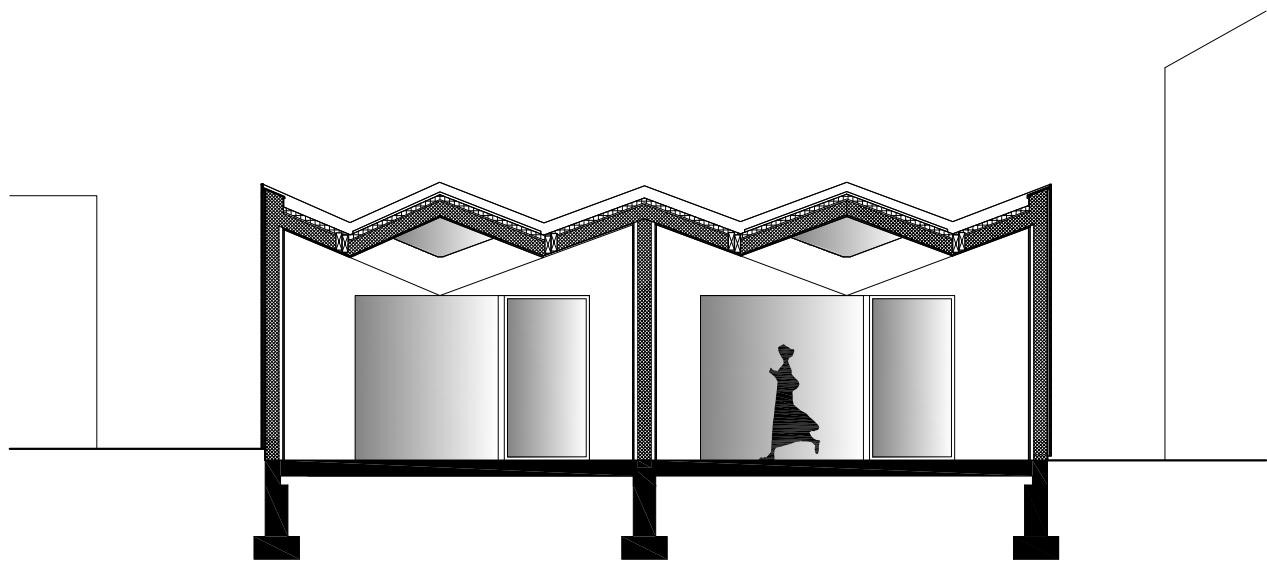
Coupe B
