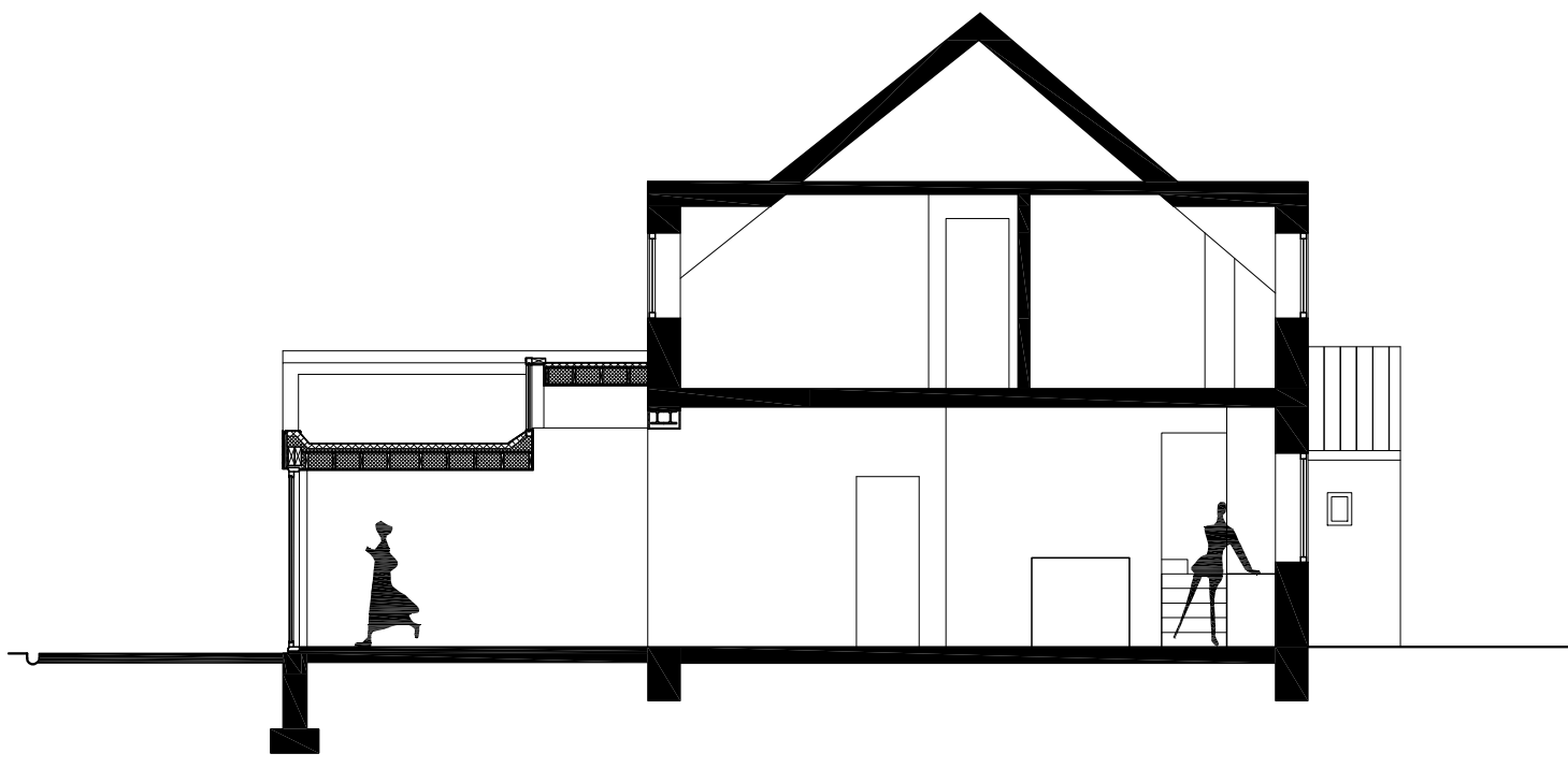
Coupe C
