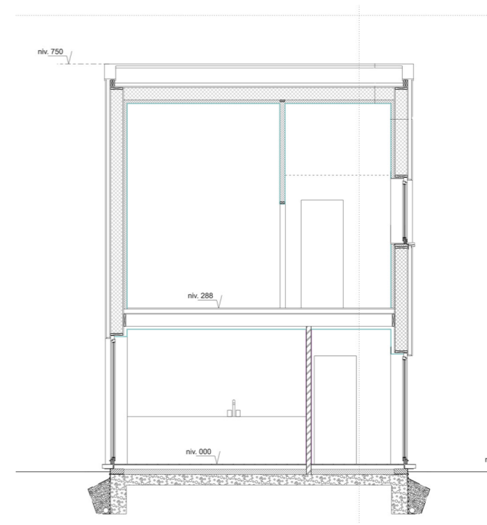
COUPE TRANSVERSALE
