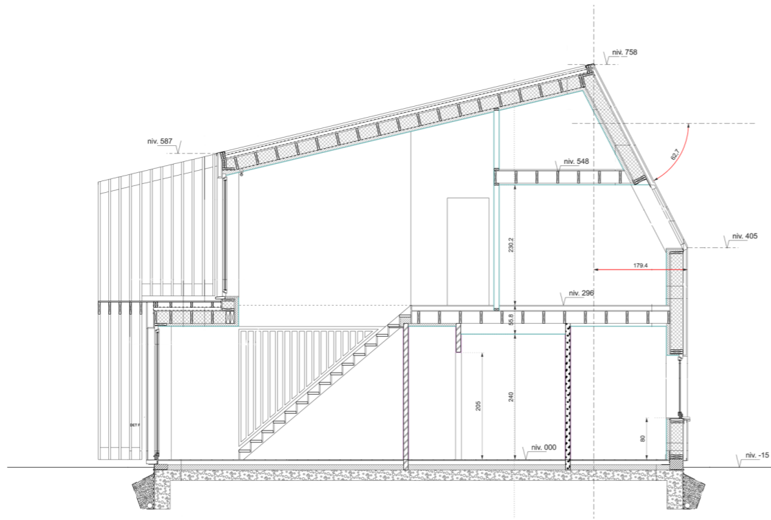
COUPE LONGITUDINALE
