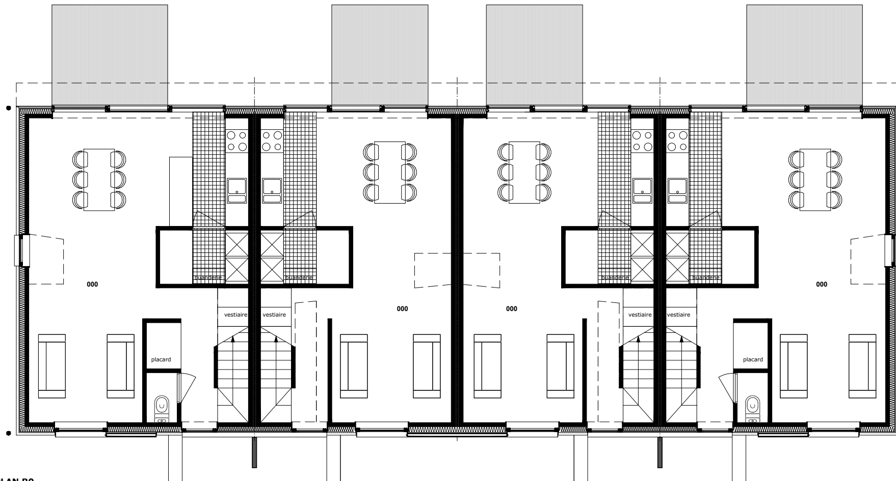
PLAN R0
