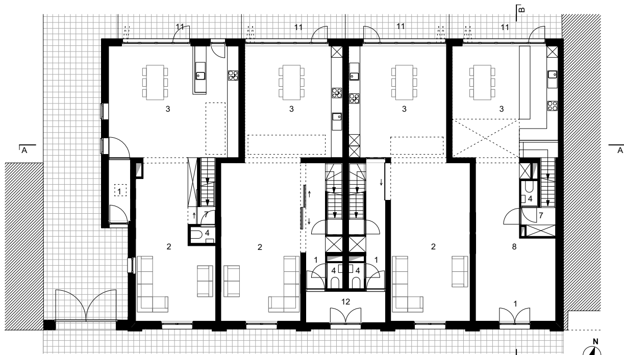
niveau 0 nieuw
