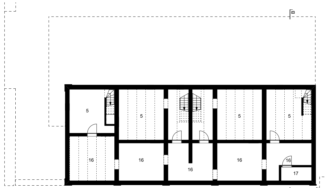
niveau -1 nieuw
