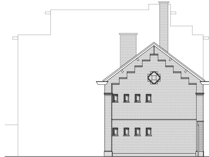
zijgevel bestaand
