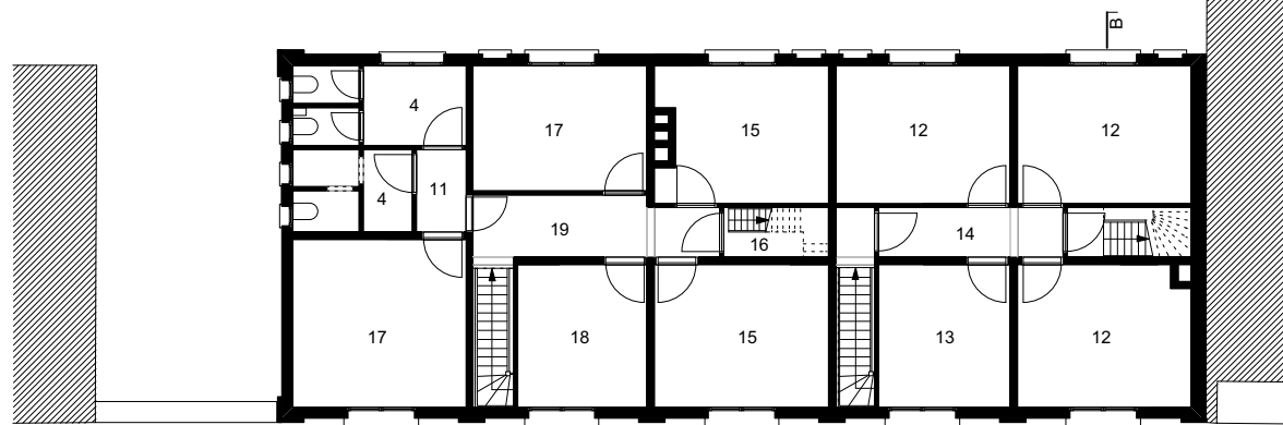
niveau 1 bestand
