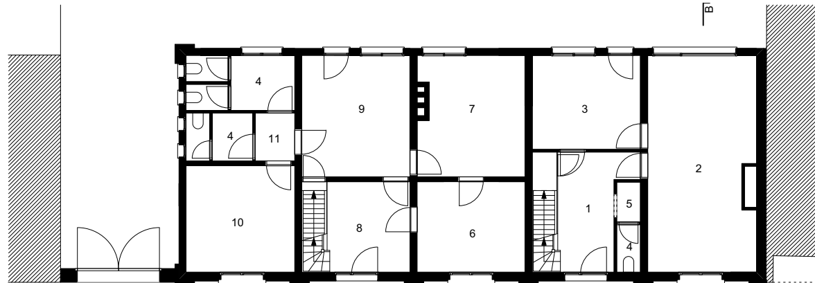
niveau 0 bestand
